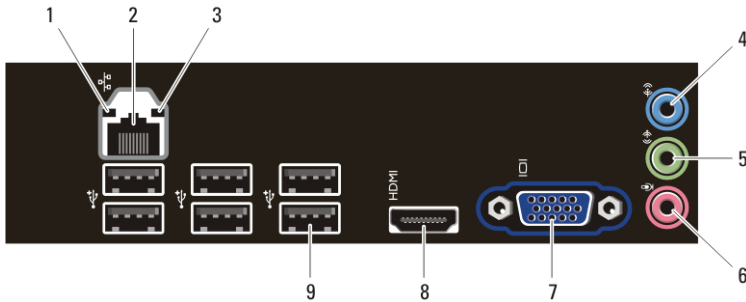
Figura 3. Vista do painel traseiro da minitorre e da torre slim
